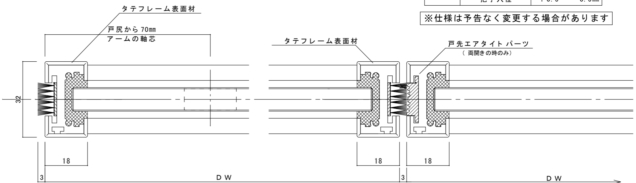
B-B断面図 S=1/1
