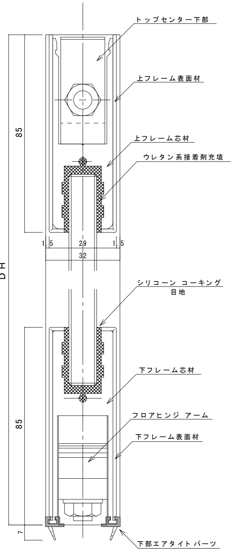
A-A断面図 S=1/1
